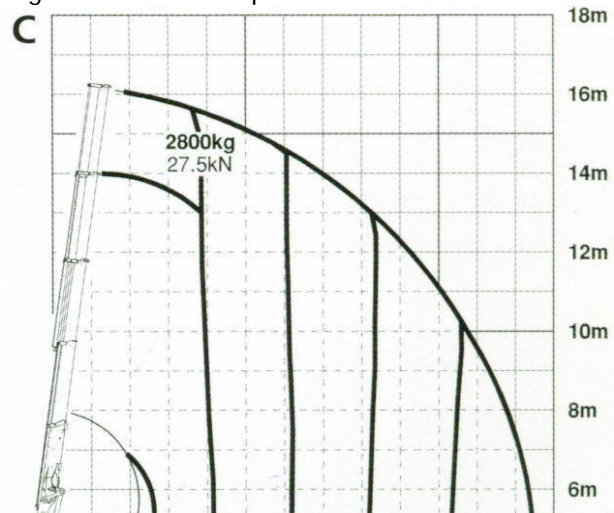
Palfinger PK20002 med spil + 3 manuelle arme
